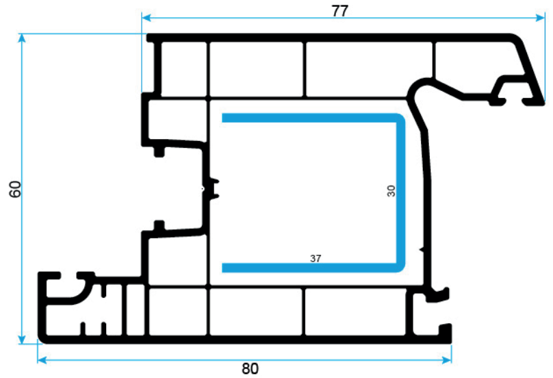
KAPI KANAT PROFİLİ DOOR SASH PROFILE
