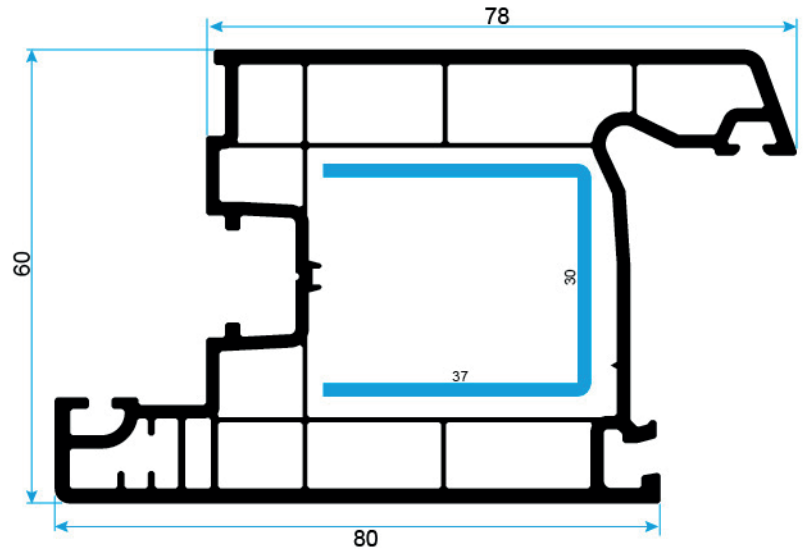
KAPI KANAT PROFİLİ DOOR SASH PROFILE
