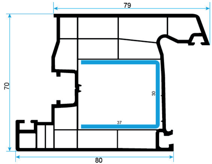
KAPI KANAT PROFİLİ DOOR SASH PROFILE
